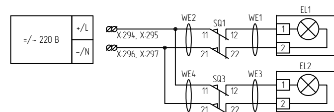
Цепи освещения шкафа
